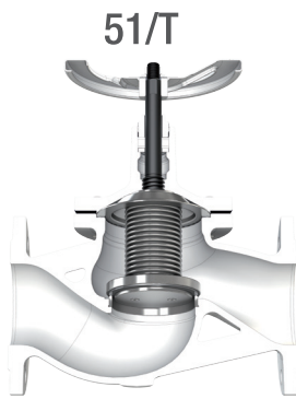
Otturatore a tenuta morbida di PTFE intercambiabile Soft sealing interchangeable PTFE disc
