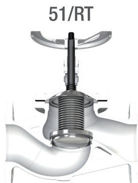
Otturatore a profilo parabolico di regolazione a tenuta morbida di PTFE intercambiabile Regulating disc with soft sealing interchangeable PTFE disc
