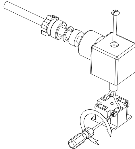
Figura 2 - Collegamento fili
