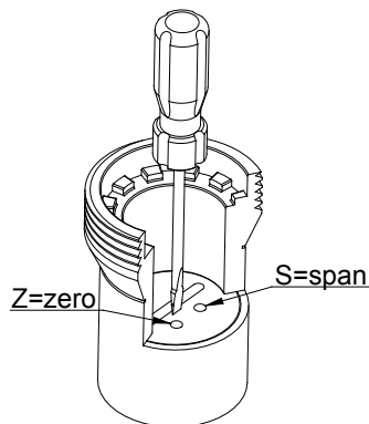
Figura 3 - Regolazione
