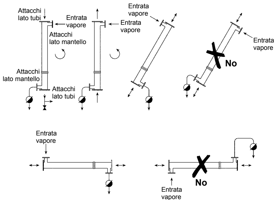
Fig. 3 - Posizionamento quando lato mantello vi sia vapore condensante
